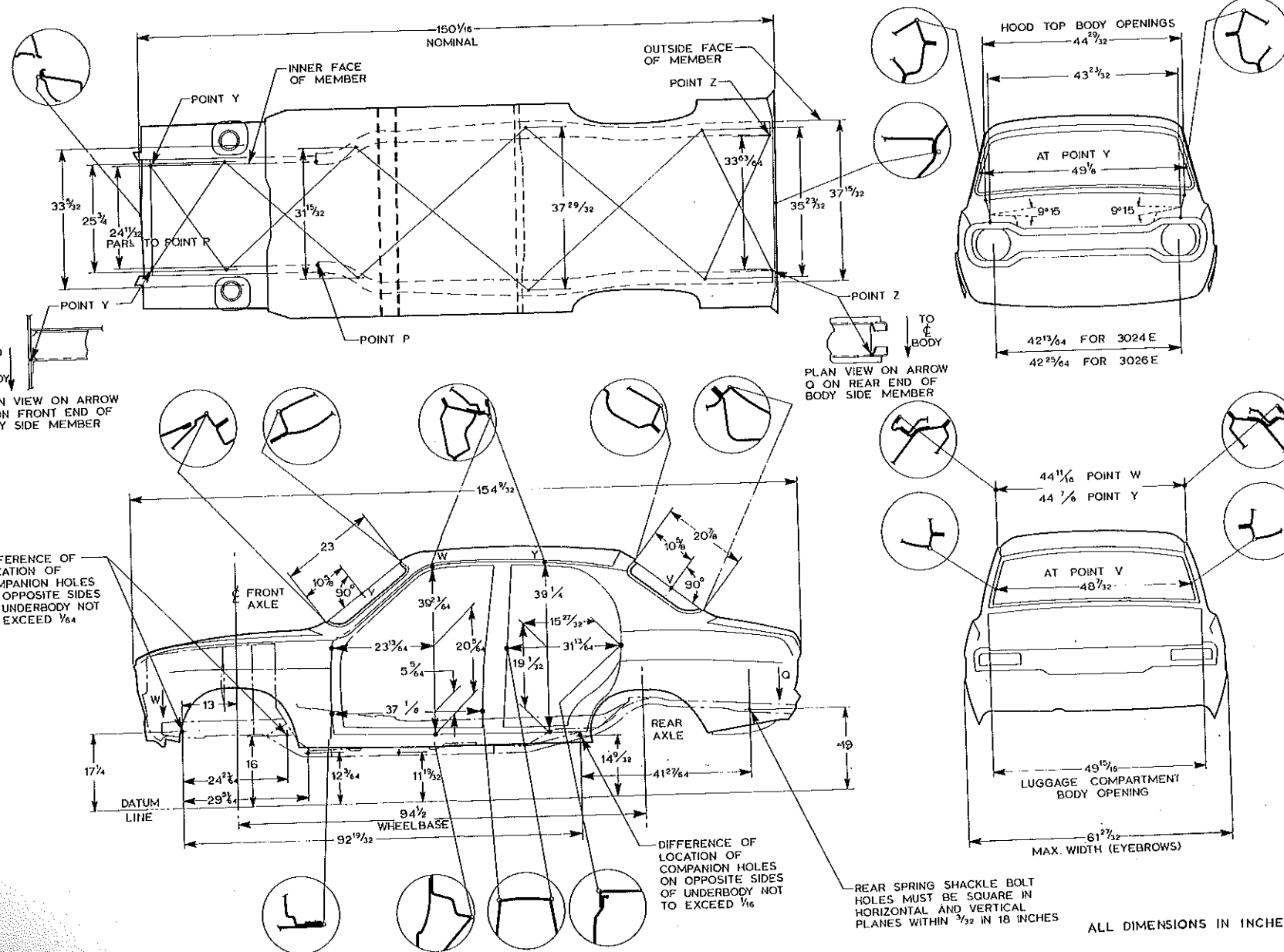
BODY TOLERANCE CHART (4 DOOR MODEL) — SEDAN
